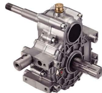
FC93风机用齿轮箱 Gear box FC93
