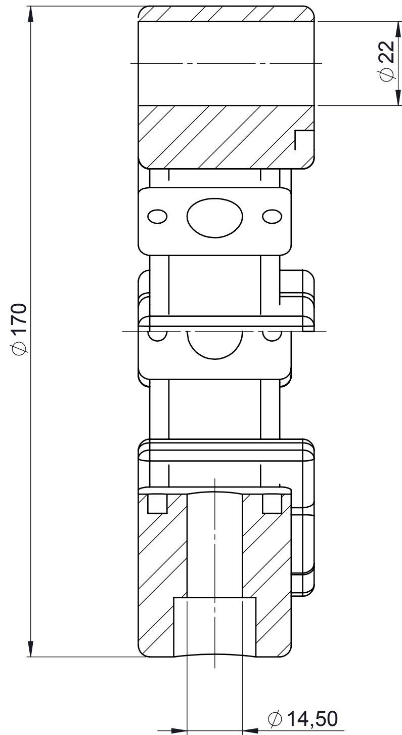
SEZIONE/SECTION A-A
